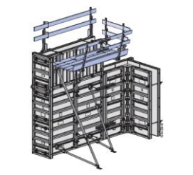
53. DOKA MURI FRAMAX
